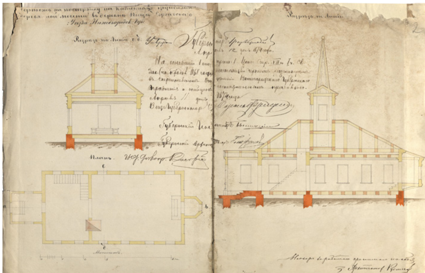
Чертеж на постройку на каменном фундаменте деревянной мечети в д. Пице Сергачского уезда Нижегородской губернии. 1874 г. ГКУ ЦАНО. Ф. 5. Оп. 1. Д. 564. Л. 1, 2.
