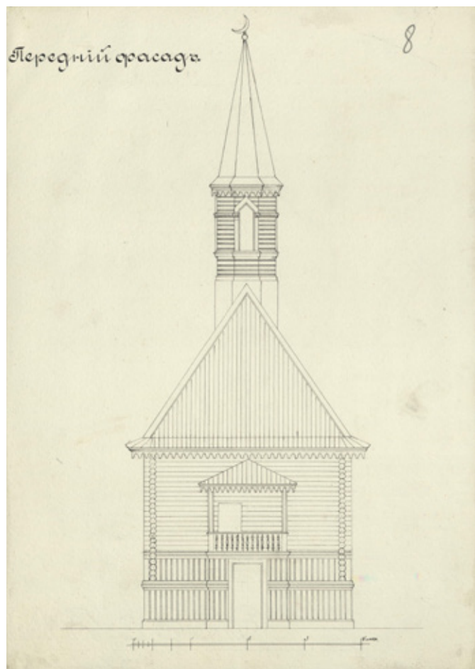
Чертеж бокового и переднего фасада мечети в д. Ишеево Андреевской волости Васильского уезда. 1902 г. ГКУ ЦАНО. Ф. 5. Оп. 50. Д. 15740. Л. 6, 8.
