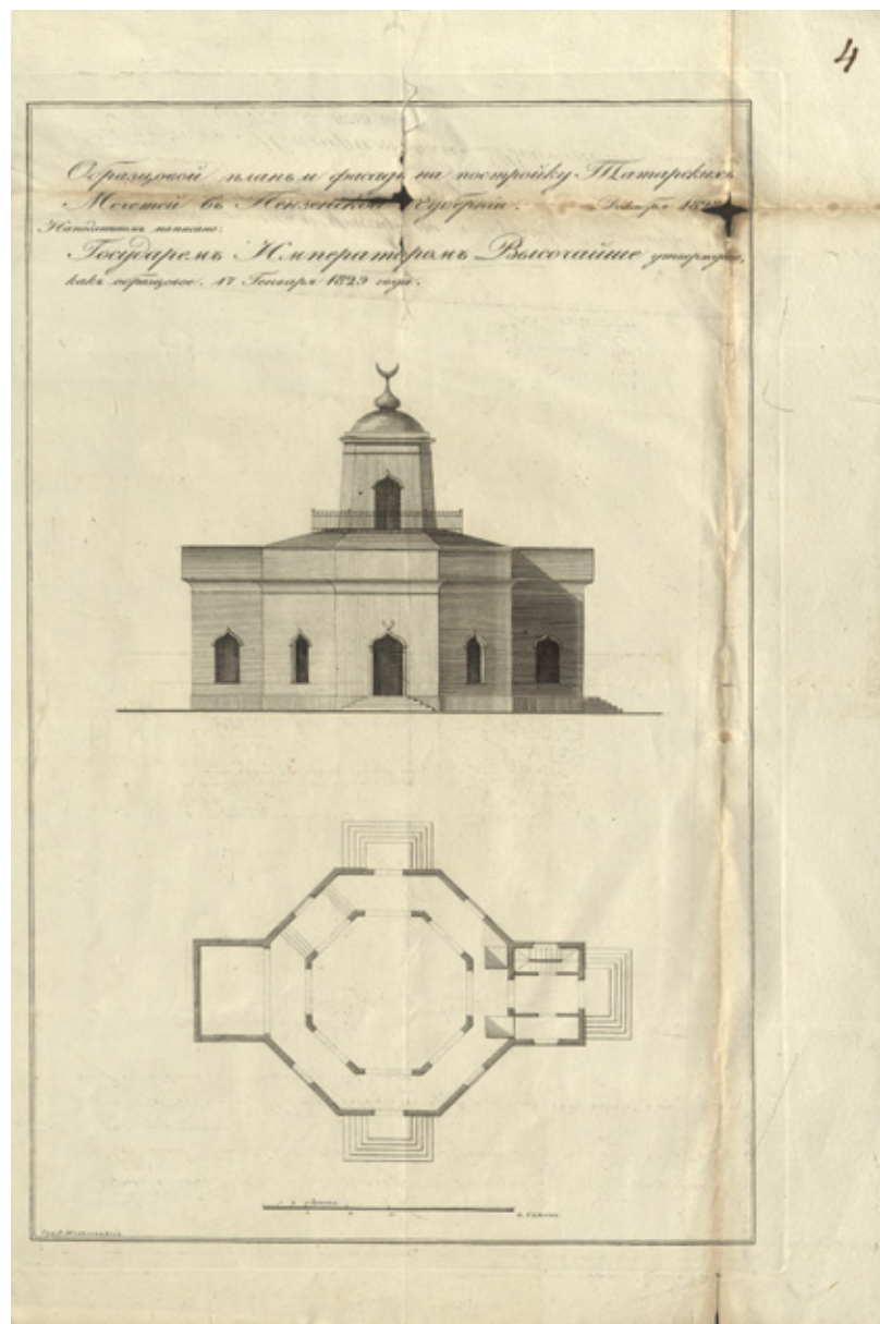
Образцовый план и фасад мечети – приложение к цирку- ляру о правилах при построении мечети. 17 января 1829 г. ГКУ ЦАНО. Ф. 2. Оп. 4. Д. 572. Л. 4.
